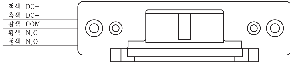
도면1 결선 방법
