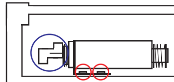
Fail Secure (정전시 닫힘) 방식
